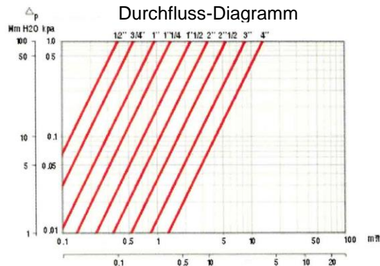
Durchfluss-Diagramm
